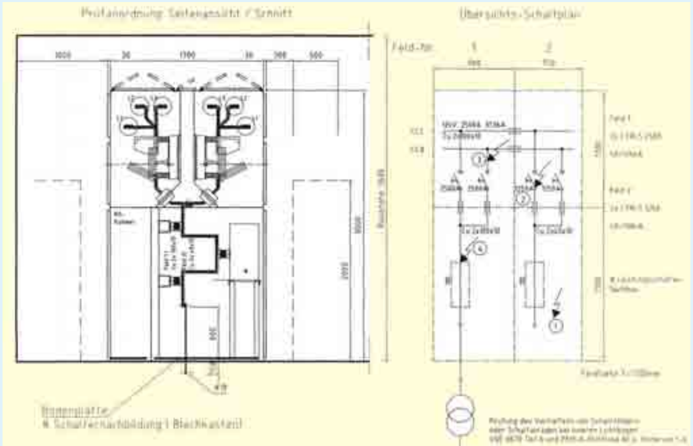
➊ Prüfanordnung (links) und Übersichtsschaltplan (rechts) der als Beispiel genannten Schaltanlage
